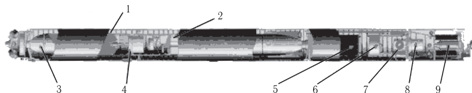
Противолодочный минно-ракетный комплекс ПМК-1
