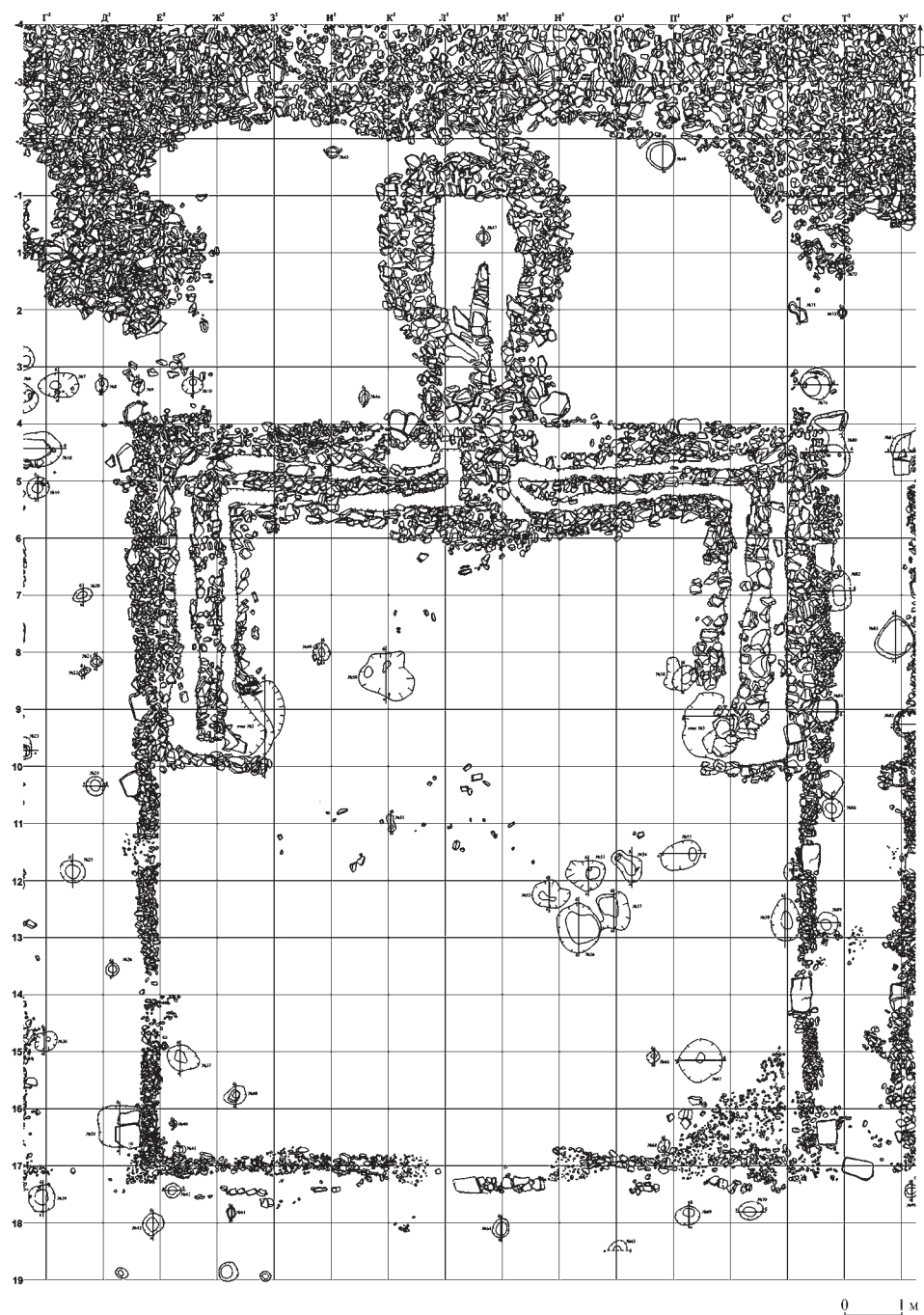
Рис. 3. План здания № 4
